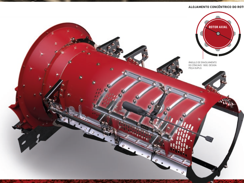
ALOJAMENTO CONCÊNTRICO DO ROTOR
